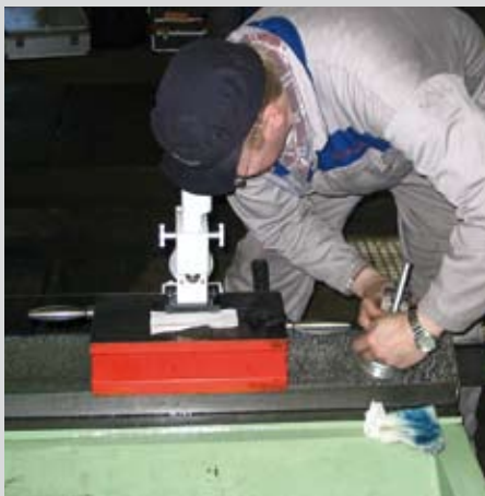
Hiomakoneen mittausta lankakäärin avulla.
